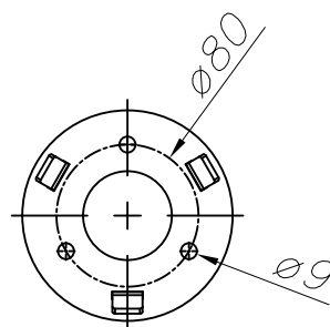
PLANTILLA DE INSTALACIÓN INSTALLATION TEMPLATE
