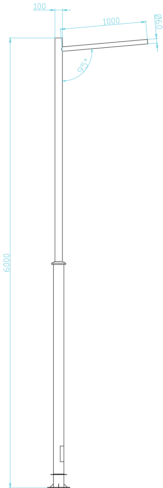
COLUMNA / COLUMN 81-4531-BP-AV
